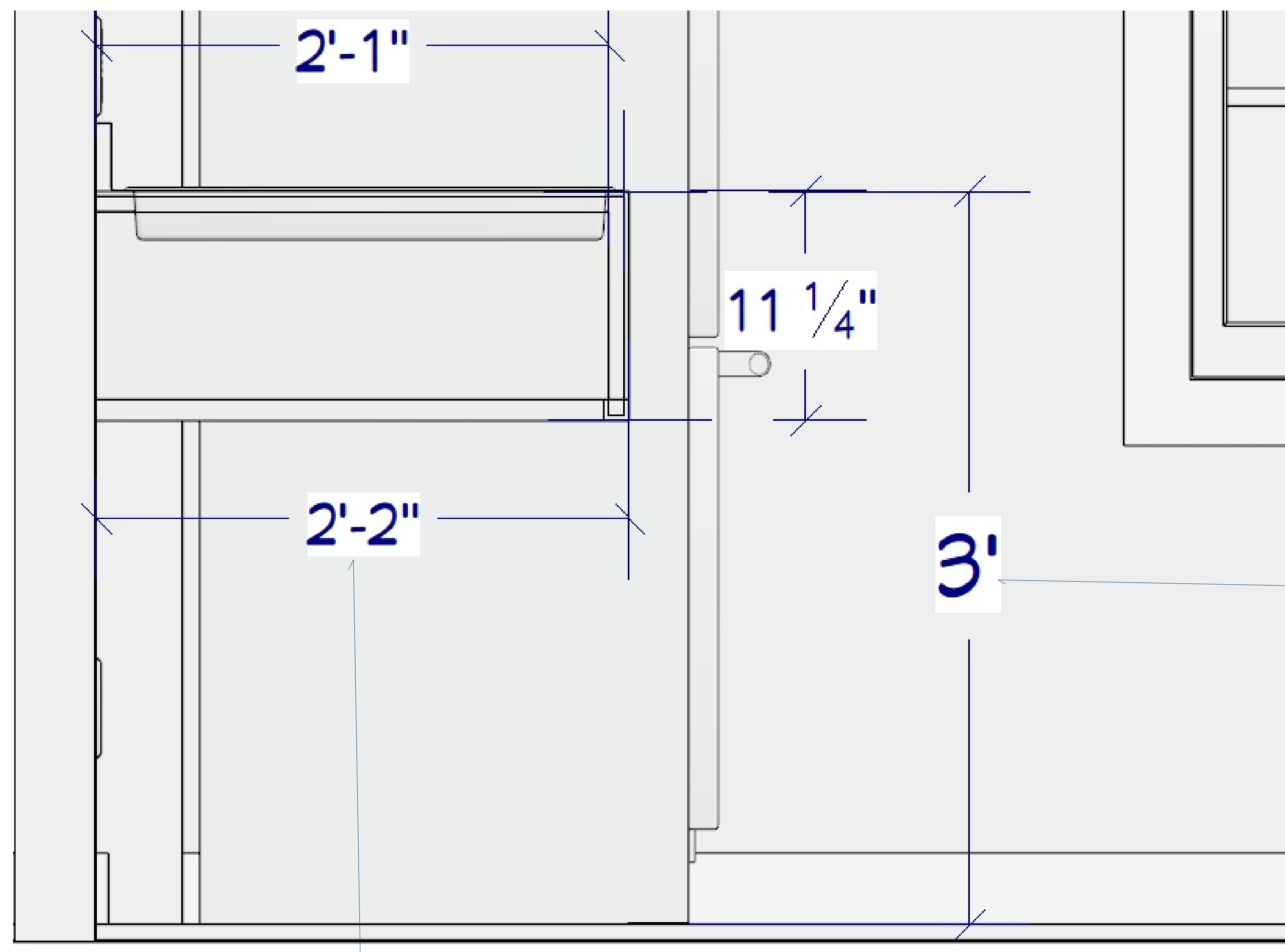
E17 A15 DIMENSIONED COUNTERTOP SECTION N.T.S.
